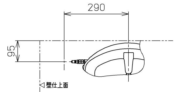
平面图
